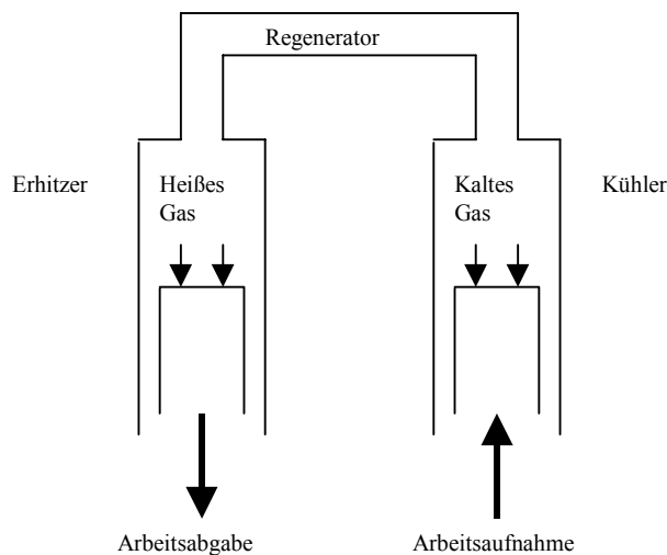
Abbildung 21 Schema eines Stirling Motors /L 35/
